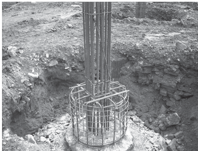
Zabetonovaná pilota protipovodňové stěny.
